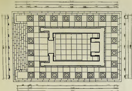
Гарни. План храма. Реконструкция А. А. Савинова
