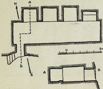
Вая. Пещерное сооружение. План.
