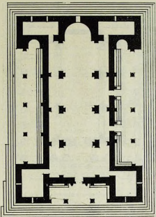
Чертеж. Триумфальная базилика, Рим.
