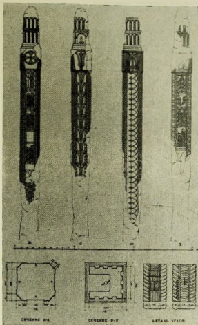
Облик Нахосских памятников Детали фасада. Обмер С. Лаврова.
