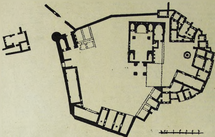
Татев. Общий план монастыря.
