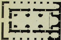
Ошун. Куольная базилика. План.
