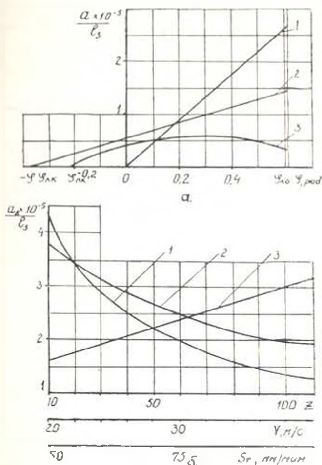
Рис. 2. а) Изменение максимальной толщины срезаемых слоев по вершинам (1), левой (2) и правой (3) сторонам нитки при нарезании колеса с z = 30 , S_t = 80 мм/мин V = 30 м/с; б) изменение максимальной толщины слоя по вершине нитки в зависимости от числа зубьев (1), скорости резания (2) и тангенциальной подачи (3).
