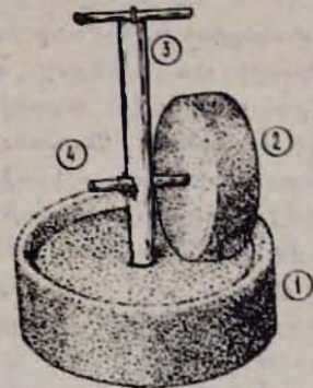
Նկ. 7. Դինգ (տինկ): 1. բարև աղաղան (կալ), 2. ուղղահայաց դարձող երկան-բաբար, 3. քարը տակի փեռների միացնող ձող (սոնի), 4. թուր:
