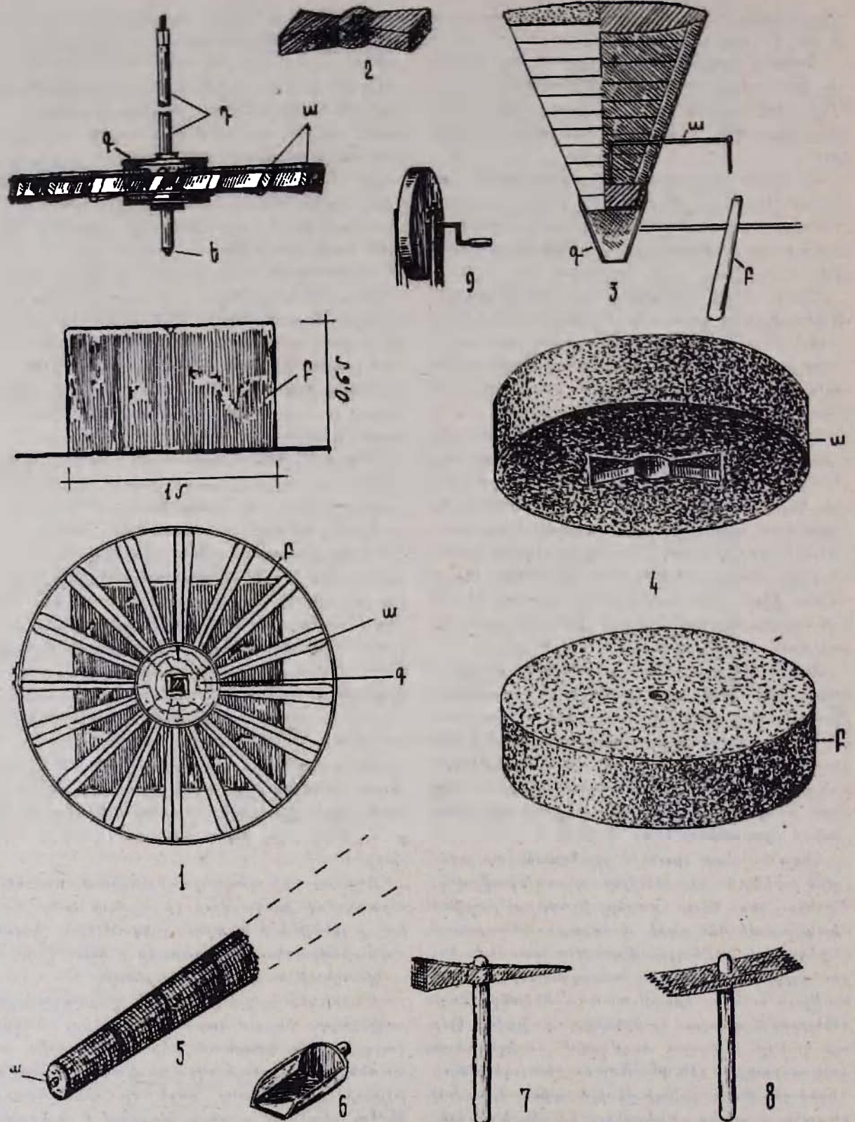
Եկ. 6. Ջրաղացի մասերը: 1. շարխ—ա. փեռի, բ. հեծնրար, գ. թուփ կամ դուռտ, դ. ստնի, Է. հե- ծան, 2. կարմուճակ, 3. համբար, 4. ջաղջըբար—ա. վրայիկեր, բ. տակիկեր, 5. նույն—ա. սիֆոն, 6. ալրաթի, 7—8. կռաններ:
