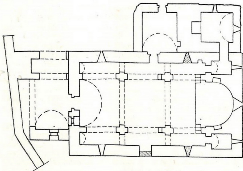
Նկ. 12բ. Հատակագիծը:
