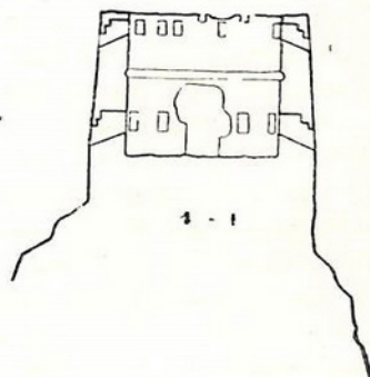
Նկ. 27ա. Մեղրու բերդը, արևմտյան կլոր աշտարակի հատակագիծը, ճակատը և կտրվածքը:
