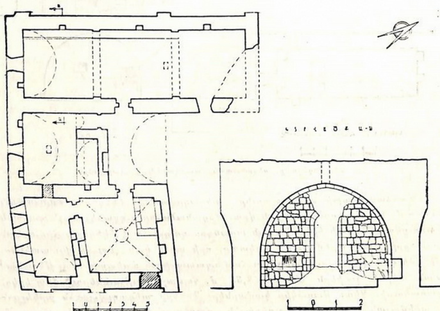
Նկ. 23. Տաթևի վանք, սեղանատան հատակադիր և կտրվածքը:
