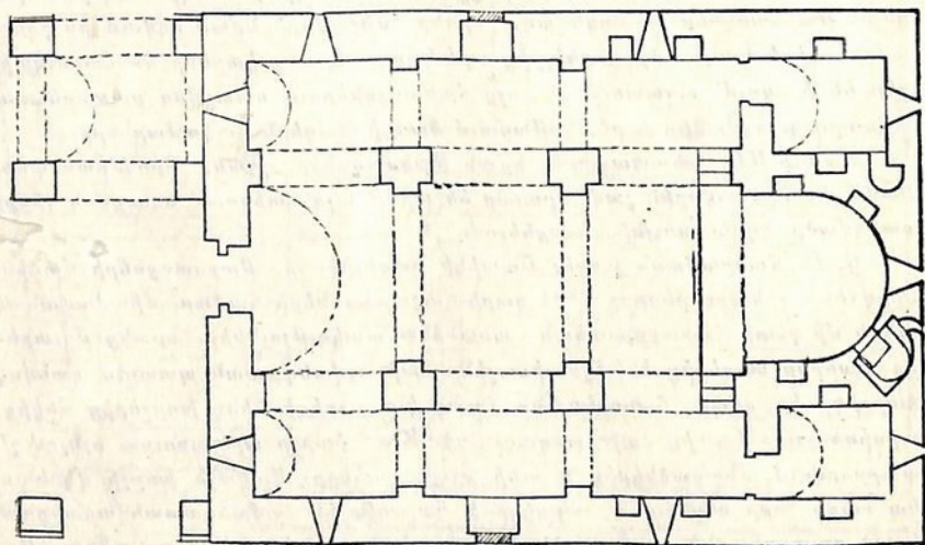
Նկ. 13բ. Հատակադիժը:
