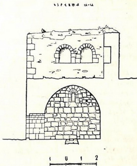
Նկ. 30. Տաթևի Մեծ անապատի. հնձանի հատակագիծը և կտրվածքը:
