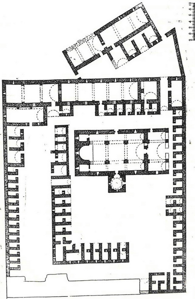
Նկ. 1. Տարբիկ Մանկ անապատ, դվանքի համալիրի ծրագիրը
