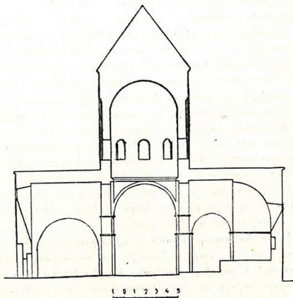
Նկ. 17ա. Մեղրու ս. Աստվածածին եկեղեցին, ընդերկայնական կտրվածքը:
