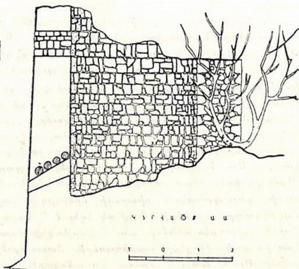
Նկ. 25բ. Բուրգի հատակադիմն ու կտրվածքը:
