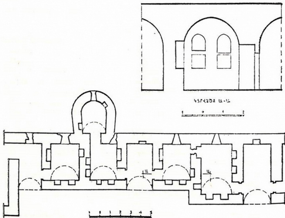
Նկ. 18. Գնդկանք, բնակելի սենյակների հատակագիծն ու կտրվածքը:
