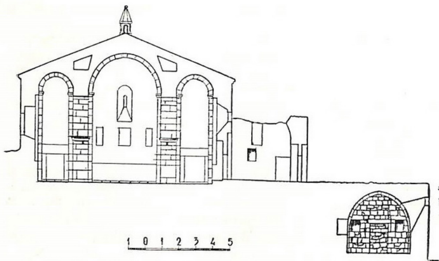
Նկ. 14ա. Շնհերի Կուսանաց անապատ, համալիրի ընդլայնական կտրվածքը:
