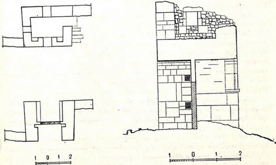
Նկ. 26. Գնդեվանք, պահակատնով դարբասի հատակագիծն ու կտրվածքը:
