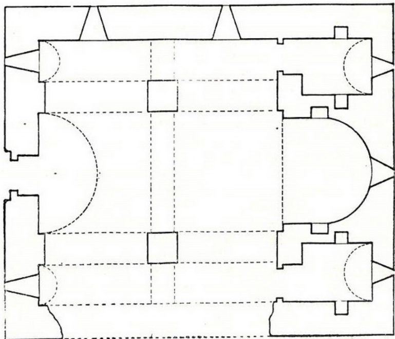
Նկ. 15. Ահեբմոնի վանքի ս. Գրիգոր եկեղեցին, ա. ընդլայնական կտրվածքը բ. հատակագիծը: 6—888
