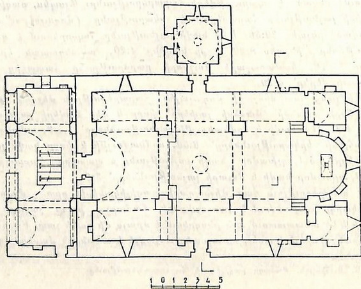
Նկ. 11բ. Հատակագիծը:
