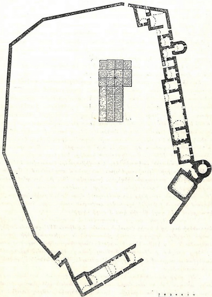
Նկ. 7. Գնդեվանք, գլխավոր հատակագիծը
