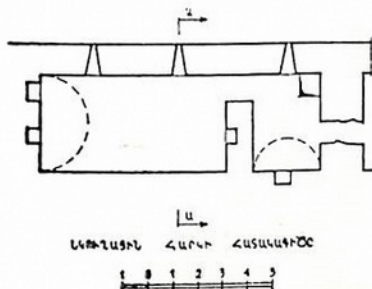
Նկ. 22. Գնդելվանք, սեղանատան հատակագիծն ու կտրվածքը:
