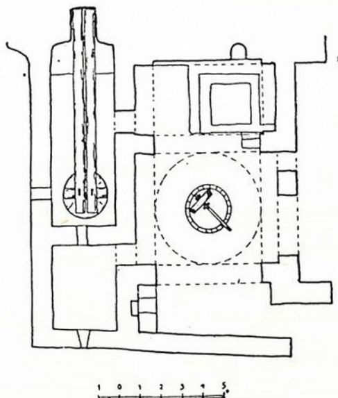
Նկ. 31. Տաթևի վանքի ձիթհանի հատակագիծը:
