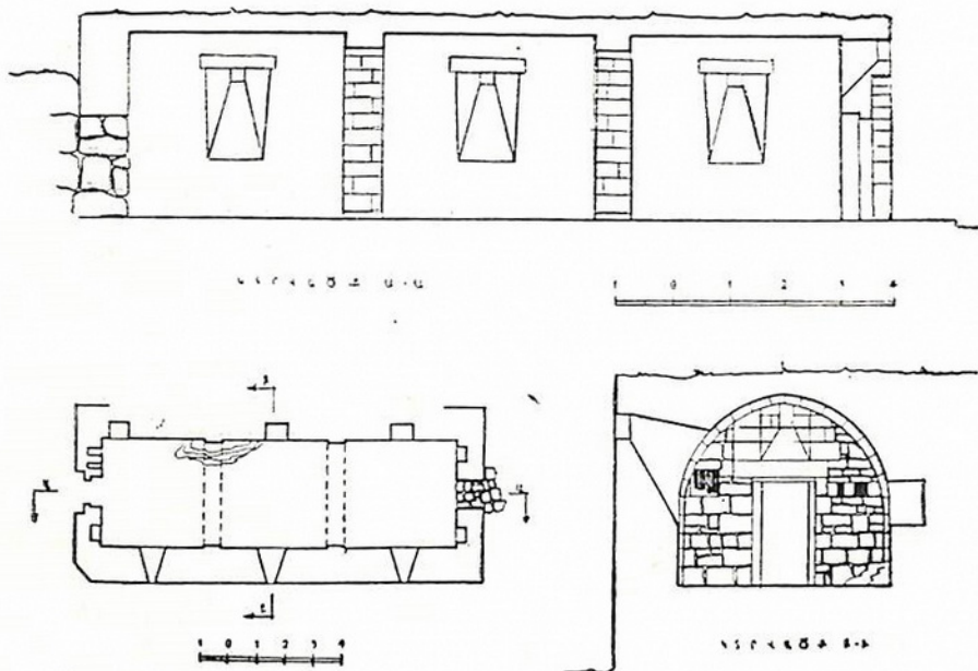
Նկ. 24. Շենհերի կուսանաց անապատ, սեղանատան հատակագիծն ու կտրվածքները:
