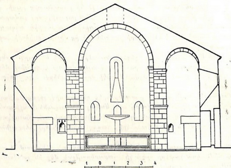
Նկ. 11ա. Տաթևի Մեծ անապատի Աստվածածին եկեղեցին, ընդլայնական կտրվածքը:
