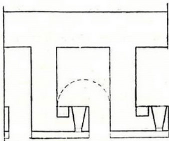
20բ. Արևմտյան և արևելյան խցերի տիպարային բլլի հատակագծերն ու ճակատները:
