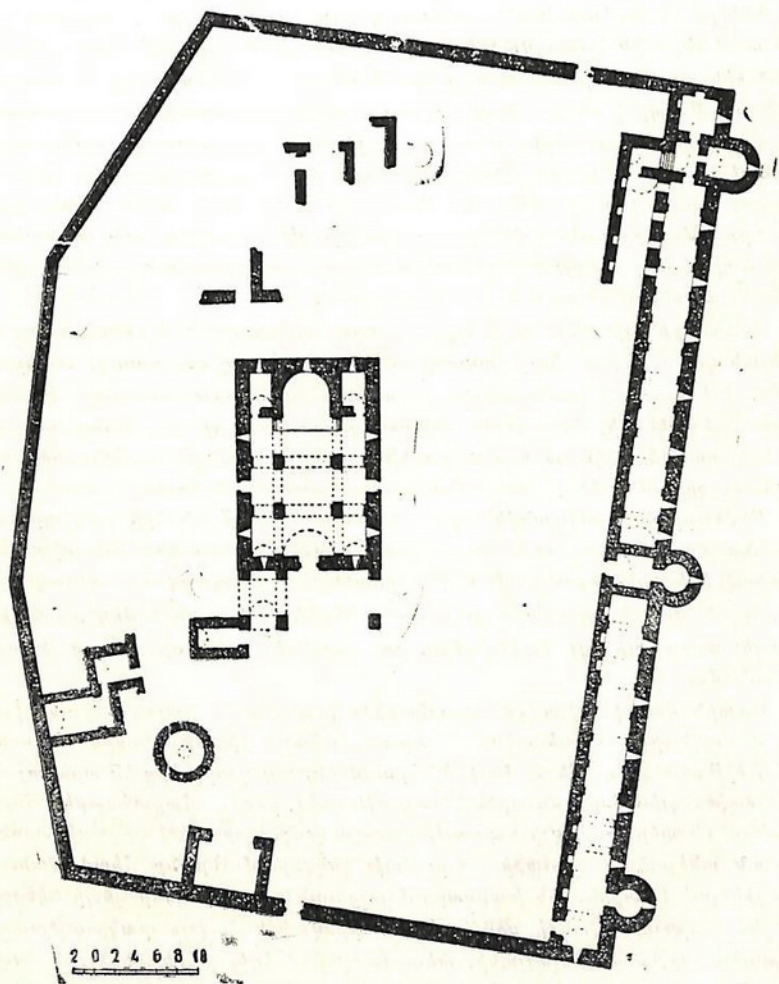
Նկ. 2. Շատին վանք, գլխավոր հատակագիծը:
