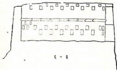
Նկ. 27ա. Մեղրու բերդը, արևմտյան կլոր աշտարակի հատակագիծը, ճակատը և կտրվածքը:
