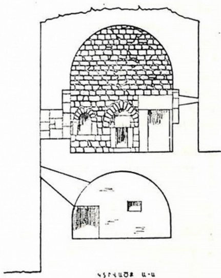
Նկ. 22. Գնդելվանք, սեղանատան հատակագիծն ու կտրվածքը:
