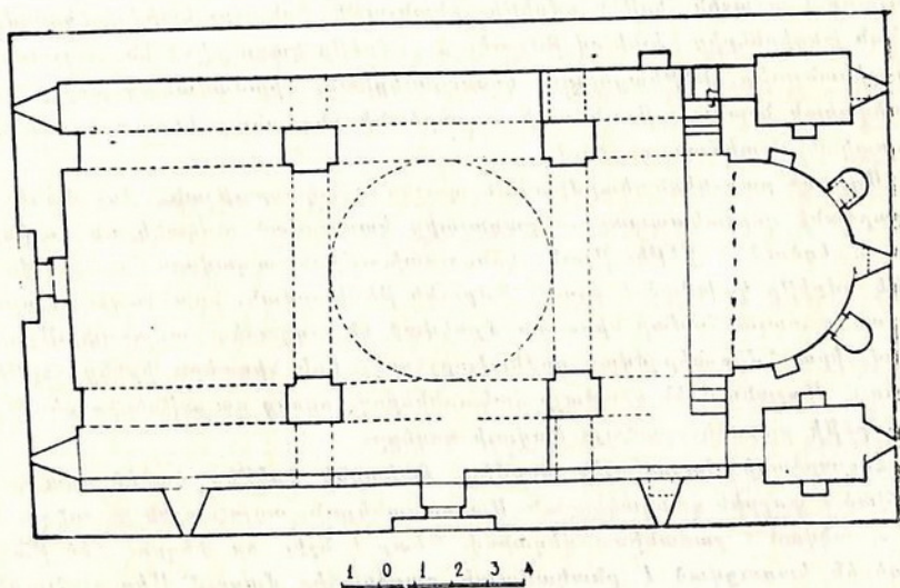
Նկ. 17բ. Հատակագիծը:
