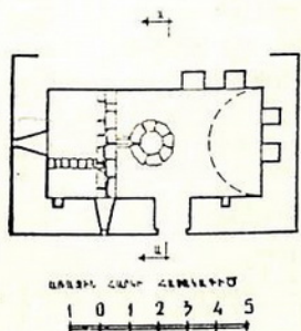
Նկ. 30. Տաթևի Մեծ անապատի. հնձանի հատակագիծը և կտրվածքը:
