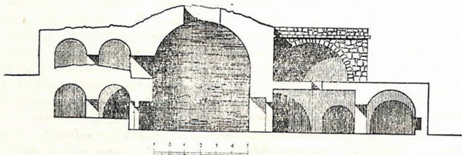
Նկ. 25ա. Հալիձորի բերդ, համալիրի կտրվածքը հյուսիսից հարավ:
