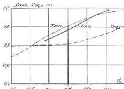
Рис. 3. Зависимости сопротивлений x_{ad3} и x_{aq3} от \alpha для генератора ECC82-4: — экспериментальная, --- расчетная.
