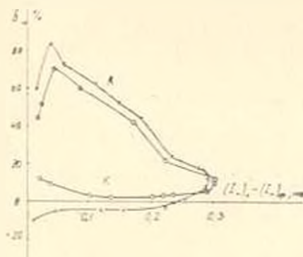
Рис. 2 Зависимость погрешности от значения выходного сигнала, вычисленная по экспериментальным данным для одного из образцов. X — случай анодной поляризации одного электрода; \square — то же другого электрода; A — при экранировании щели анодом; K — то же катодом.
