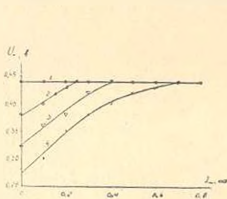
Рис. 3. Зависимость выходного сигнала при фотоэлектрическом считывании от переменного тока с f = 100 цз, наложенного на ток управления: 1 — I_0 - I_n = 0 ; 2 — I_0 - I_n = 0,05 мА; 3 — I_0 - I_n = 0,1 мА; 4 — I_0 - I_n = 0,15 мА
