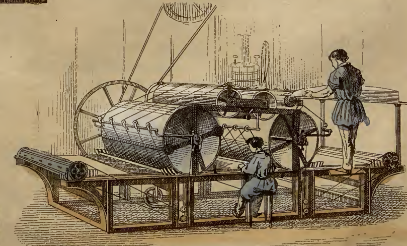
19. Presse Mécanique, mue par la Vapeur.
