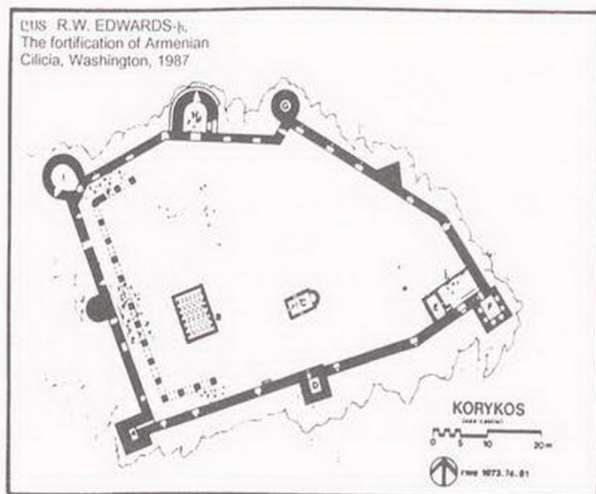
Գծագիր 9. Կորիկոս ամրոցի չափագրությունը ըստ Ռ. Վ. Էդվարսի, 1981 թ.:
