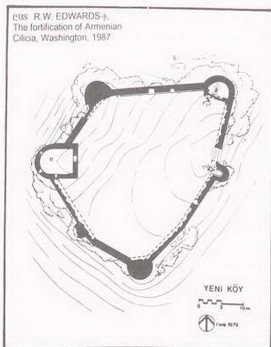
Գծագիր 8. Յենի Կյոյ ամրոցի չափագրությունը ըստ Ռ. Վ. Էդվարսի, 1979 թ.:
