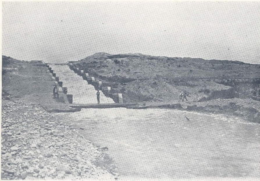
ՓՈՒՐ ՍԱՐԿԱՐԱՐԱՏԻ ՈՌՈՒՄԱՆ ՍԻՍՏԵՄԻ ԶՐԹԱՓԸ
