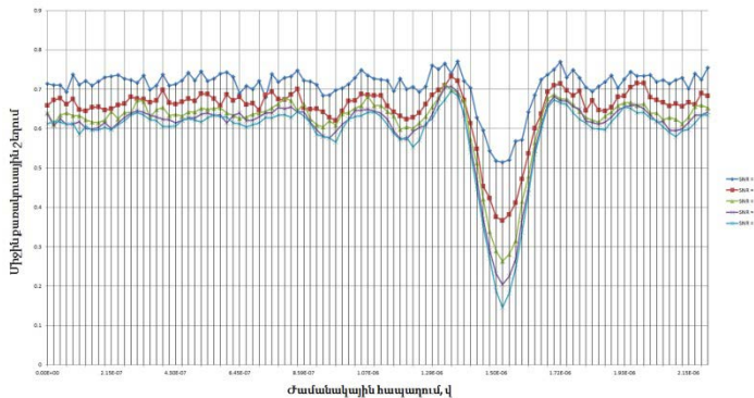
Նկ. 5. Միջին քառաձուսային շեղման կախվածությունը ժամանակային հապաղման գտման քայլից, տարբեր մակարդակի գաուսյան աղմուկների դեպքում
