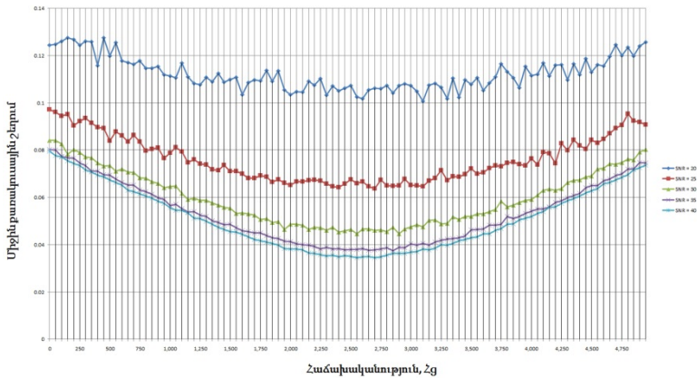
Նկ. 9. Միջին քառակուսային շեղման կախվածությունը դրվերյան հաճախականային շեղման գտման քայլից, տարբեր մակարդակի գաուսյան աղմուկների դեպքում
