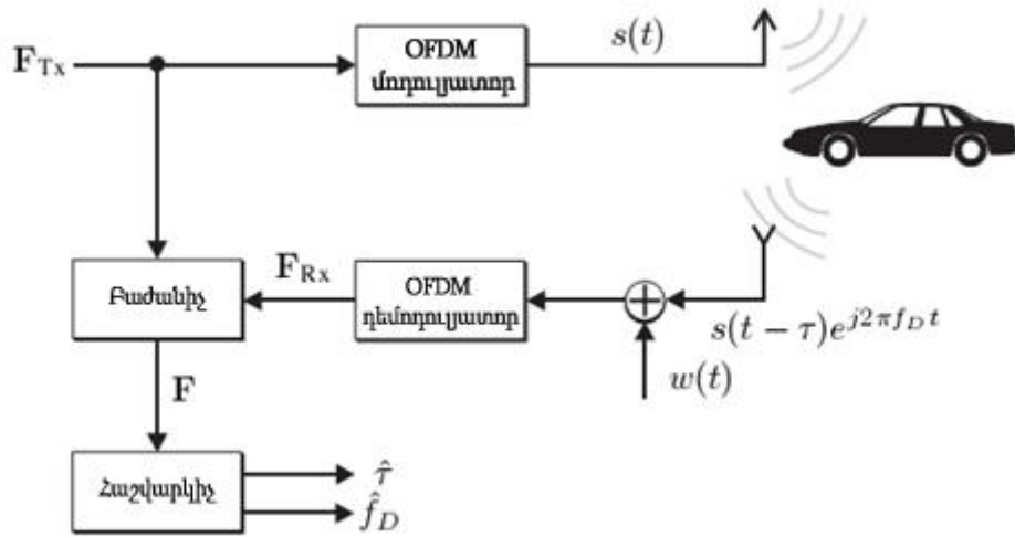
Նկ. 1.3.3. Ներկայացված OFDM ուղիղորկացիոն համակարգի աշխատանքը:
