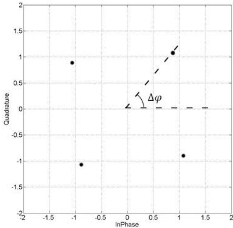
Նկ. 3.3.5. Q սիմվոլների միջինացված համաստեղությունը, ժամանակային հապաղման առկայության դեպքում:
