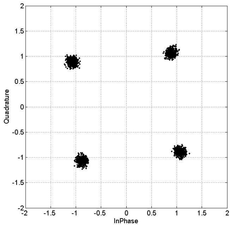
Նկ. 3.4.1. Դոպլերյան շեղմամբ OFDM ազդանշանի համաստեղությունը՝ մինչև միջինացման իրականացումը:
