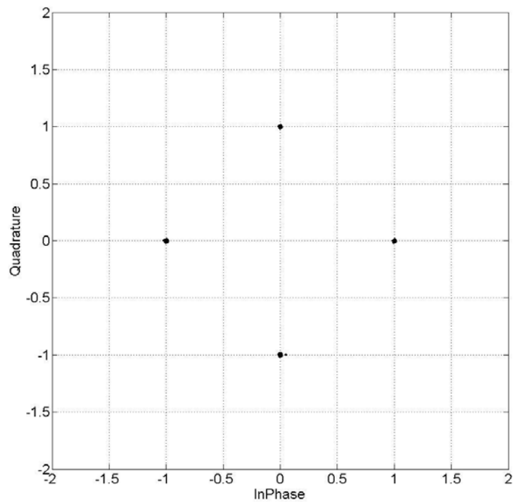
Նկ. 3.3.2. Հարևան ենթակրողների հարաբերությամբ ձևավորված, նոր՝ Q սիմվոլների համաստեղությունը՝ աղավաղումների բացակայության դեպքում:
