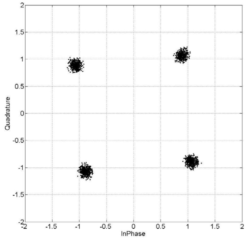
Նկ. 3.1.6. Շարժվող թիրախից անդրադարձած OFDM ազդանշանի համաստեղությունը՝ զտված \tau_3 = 143\Delta\tau = 1.54\mu\text{վ} հապաղմամբ:
