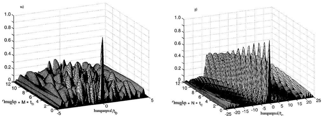
Նկ. 1.3.6. M \times M չափանի MCPC(w) և M^2 չափանի P4(p) ազդանշանների անորոշության ֆունկցիաները:
