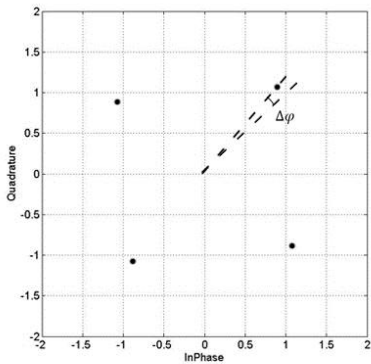
Նկ. 3.4.2. Դոպլերյան շեղմամբ OFDM ազդանշանի համաստեղությունը միջինացման պրոցեսինգ հետո:
