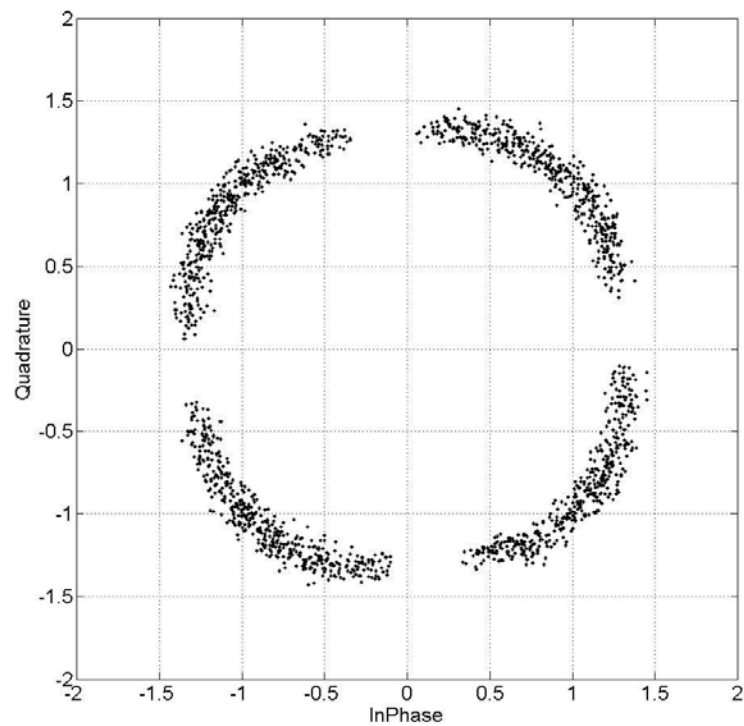
Նկ. 3.1.7. Շարժվող թիրախից անդրադարձած OFDM ազդանշանի համաստեղությունը՝ զտված \tau_4 = 147\Delta\tau = 1.58\mu\text{վ} հապաղմամբ:
