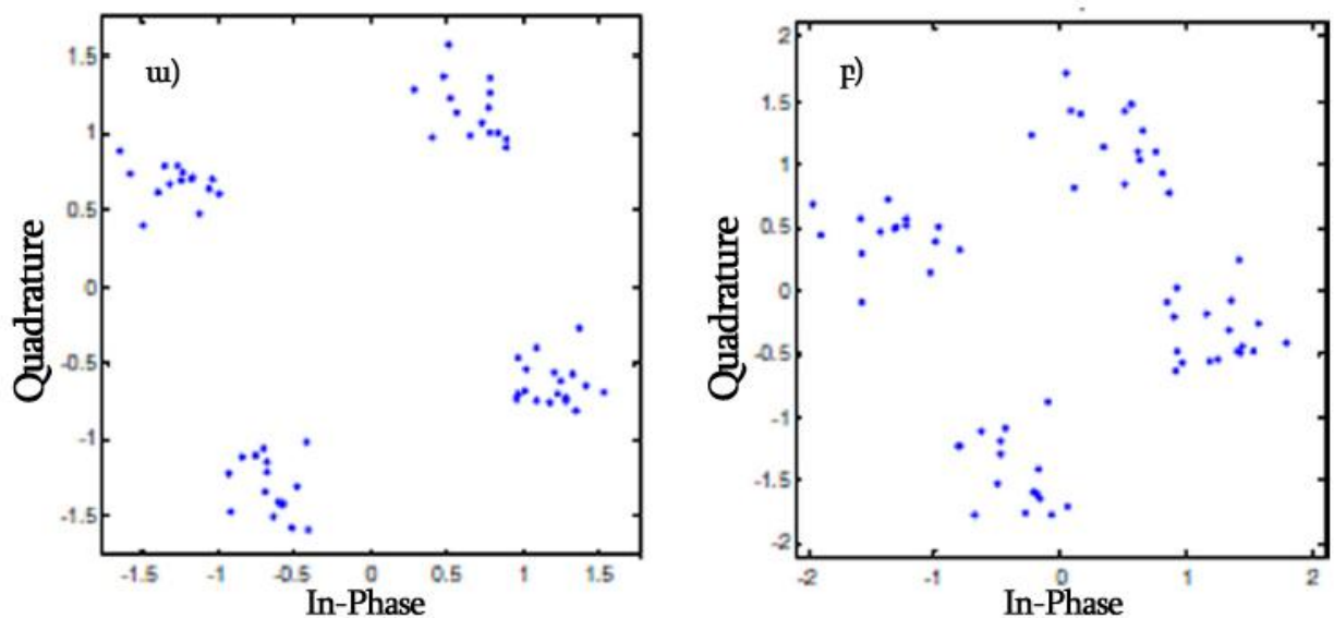
Նկ. 1.3.7. Տարբեր CFO-ի ազդեցությամբ(30%Հց(ա), 50%Հց(բ)) OFDM արձագանք-ազդանշանի կոնստելացիան:
