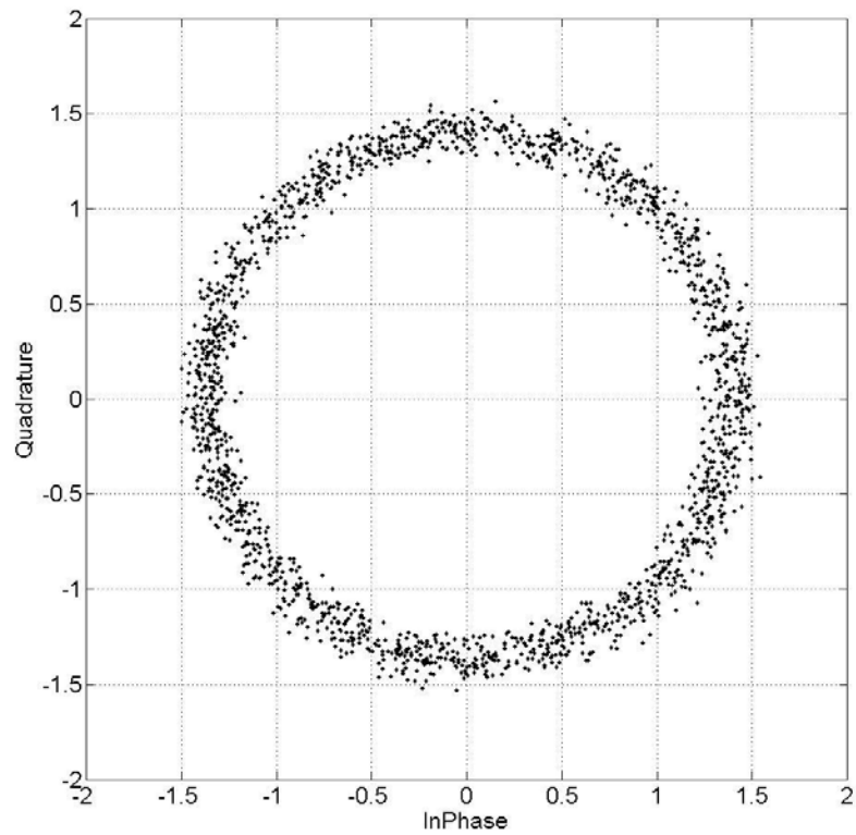
Նկ. 3.1.4. Շարժվող թիրախից անդրադարձած OFDM ազդանշանի համաստեղությունը՝ գտված \tau_1 = 100\Delta\tau = 1.07\mu\text{վ} հապաղմամբ:
