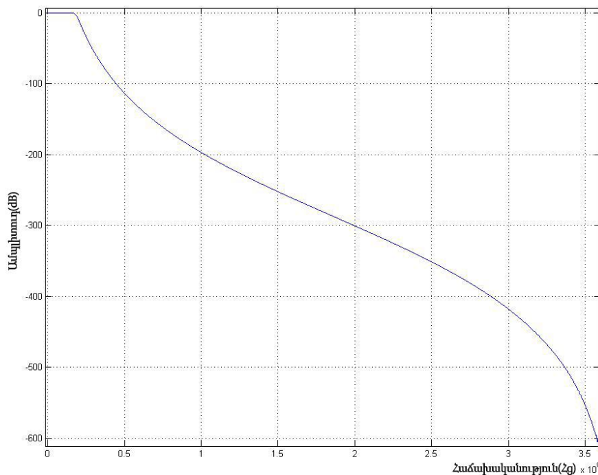
Նկ. 2.1.6. Թվա-անալոգային բատերֆորդյան գոծիչի բնութագիրը:
