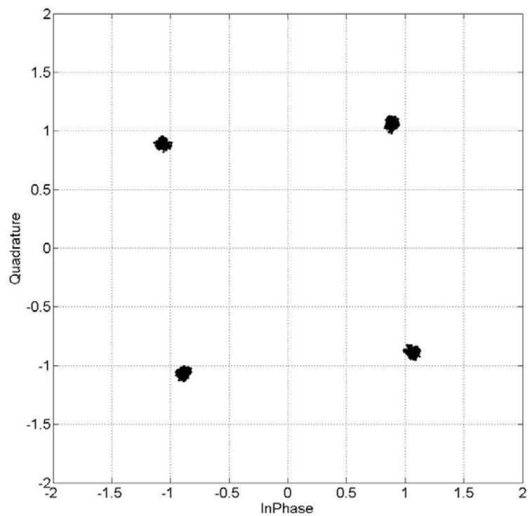
Նկ. 3.3.4. Հարևան ենթակրողների հարաբերությամբ ձևավորված, նոր՝ Q սիմվոլների համաստեղությունը, ժամանակային հապաղման առկայության դեպքում:
