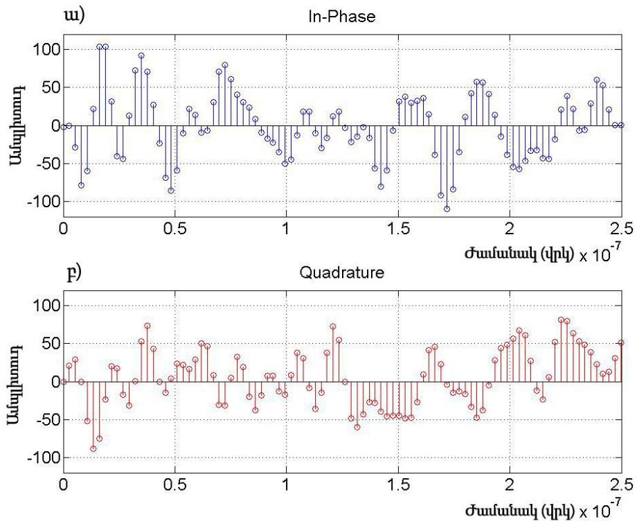
Նկ. 2.1.16. Ընտրությամբ վերականգնված OFDM ազդանշանի ժամանակային բնութագիրը. In-Phase բաղադրիչը (ա)-ում, Quadrature բաղադրիչը (բ)-ում:
