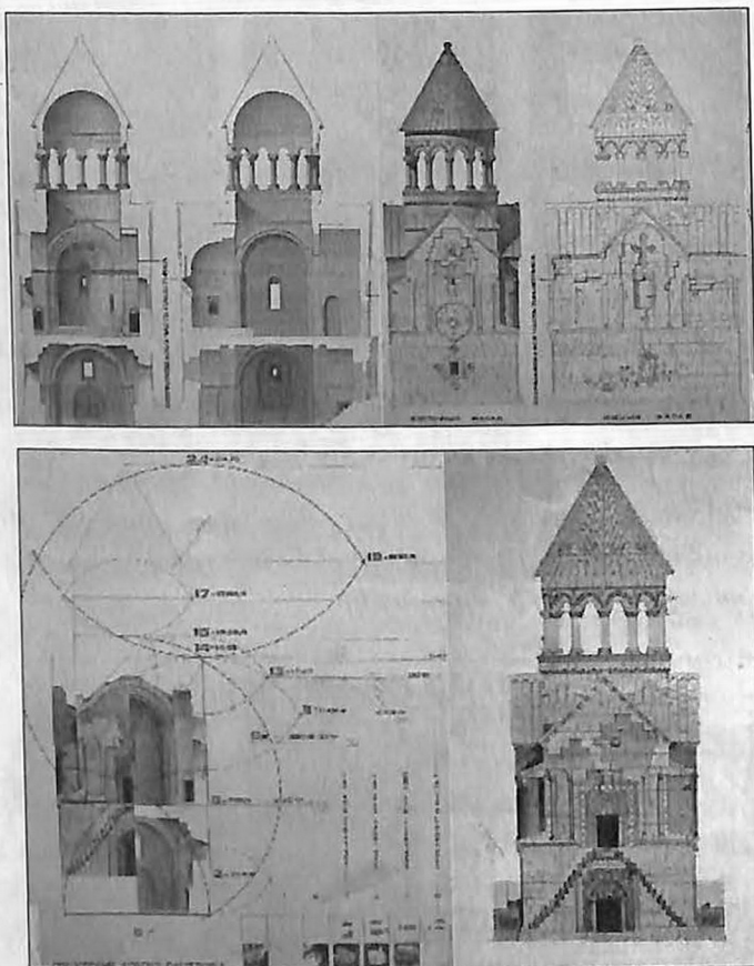
Նորավանքի Բուրթելաշէն եկեղեցու վերականգնման նախագիծ
