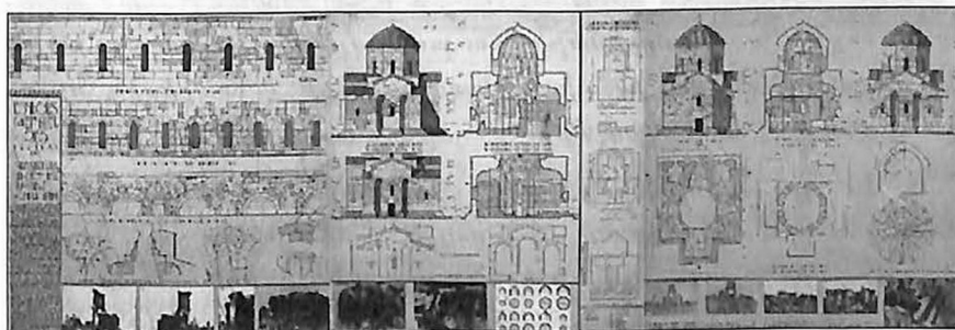
Այգեշատի Թարգմանչած եկեղեցու վերականգնման նախագիծ 77
