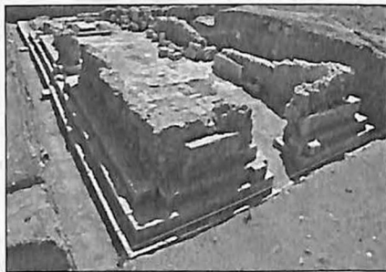
Նկար 5. Արցախի Տիգրանակերտի վաղճրիստոնեական եկեղեցին (1) եւ արտաքին ջրահեռացման համակարգը (2)
