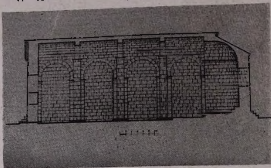
ՄԱՅՐ ՏԱՃԱՐԻ Դ ԴԱՐԻ ԿԱՌՈՒԹՎԱԾՔԻ ԸՆԴԵՐԿԱՅՆԱԿԱՆ ԿՏՐՎԱԾՔԻ ՎԵՐԱԿԱՋՄՈՒԹՅԱՆ ՆԱԽԱԳԻԾԸ
