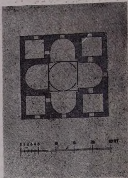
ՄԱՅՐ ՏԱՃԱՐԻ ՀԱՏԱԿԱԳԻԾԸ ԸՍՏ Թ. ԹՈՐԱՄԱՆՑԱՆԻ ՎԵՐԱԿԱՋՄՈՒԹՅԱՆ
