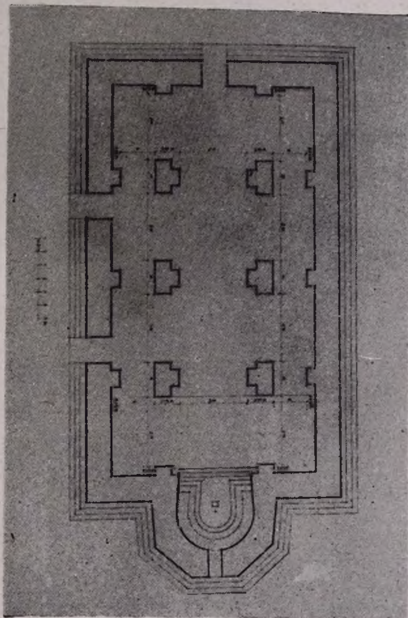
ՄԱՅՐ ՏԱԺԱՐԻ Դ ԴԱՐԻ ԿԱՌՈՒՑՎԱԾԻ ՀԱՅԿԱՎԱԳՈՒ ՎԵՐԱԿԱԶՄՈՒԹԱՆ ՆԱԽԱԳԻԾԸ
