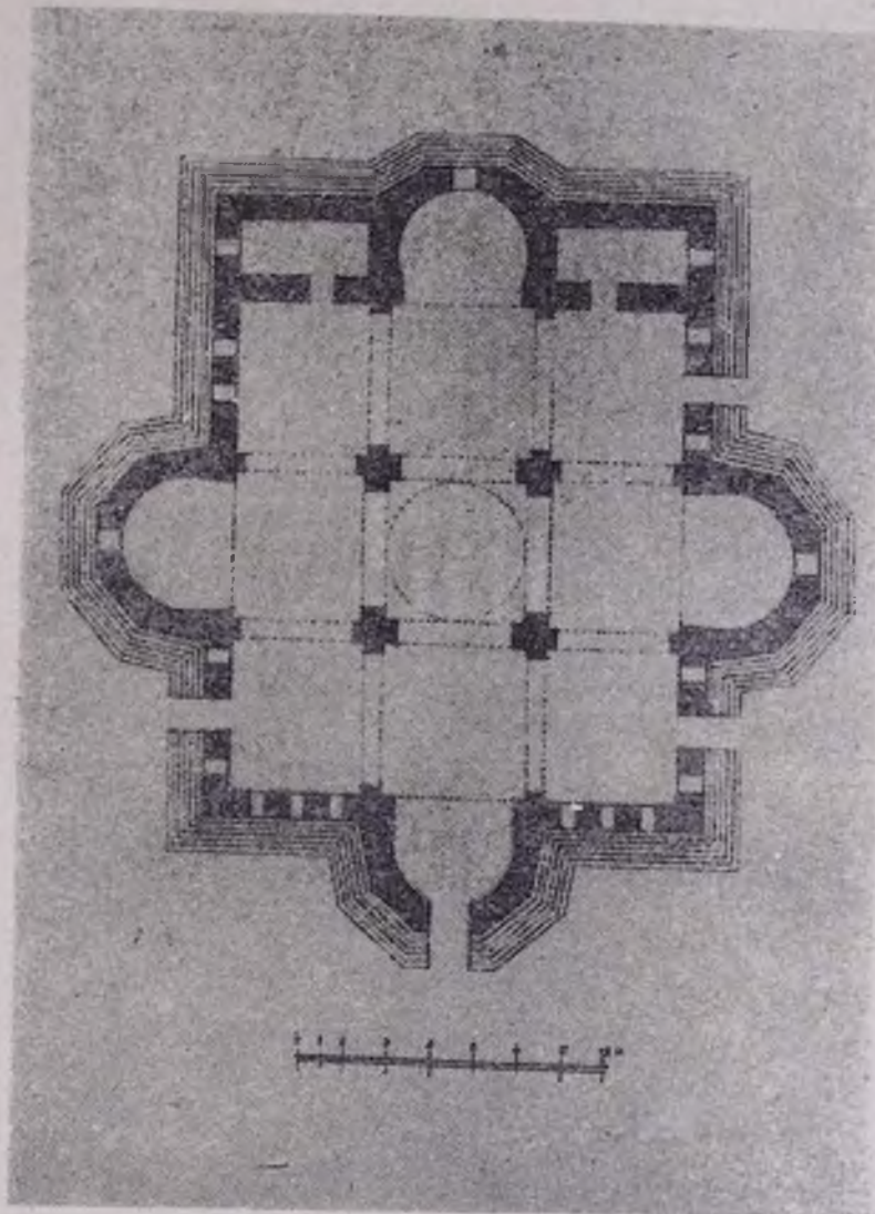
ՄԱՅՐ ՏԱՃԱՐԻ Ե ԴԱՐԻ ԿԱՌՈՒԹՎԱԾՔԻ ՀԱՅԱԿԱՐԳԻՄԸ
