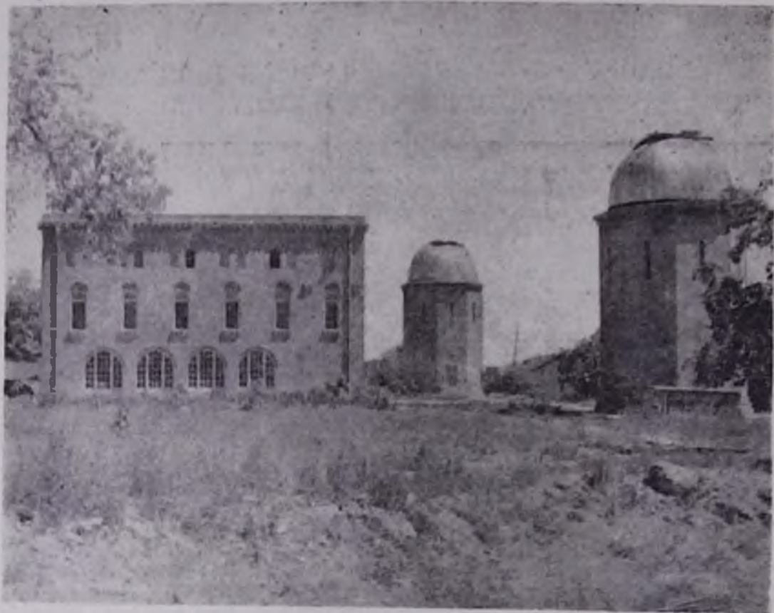
Սյուրականի աստղադիտարանը
