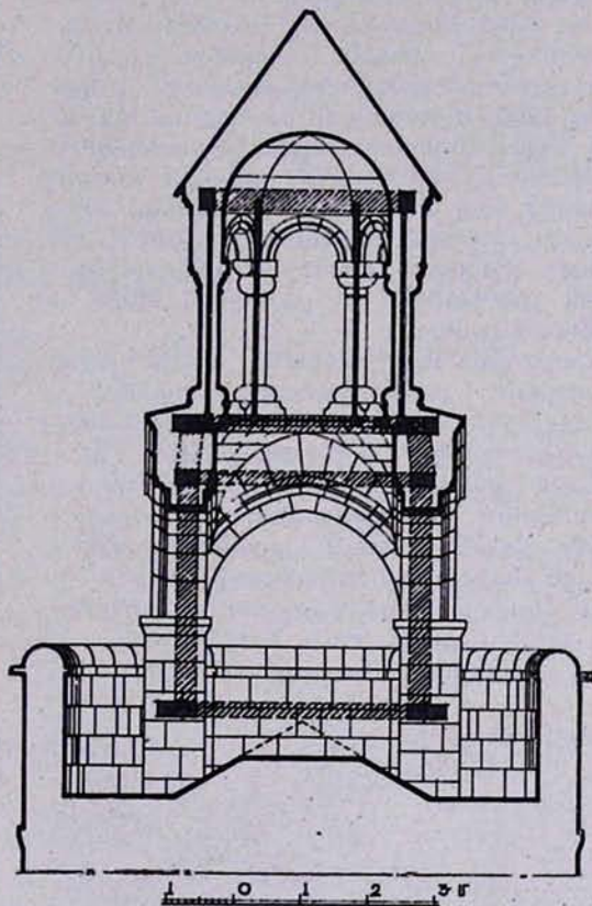
Նկ. 2. Հարավային զանգակատան վերականգնման կոնստրուկտիվ գծագիրը
