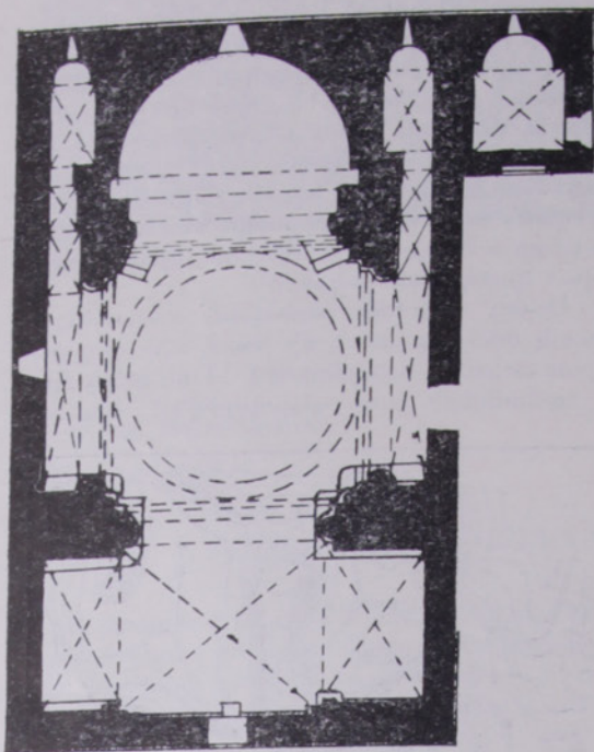
Նկ. 2. Աստվածածին եկեղեցու հատակագիծը
