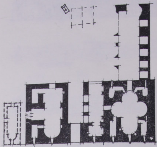
Նկ. 1. Ցախազքար վանք.—Արևմտյան խմբի ընդհանուր հատակագիծը
