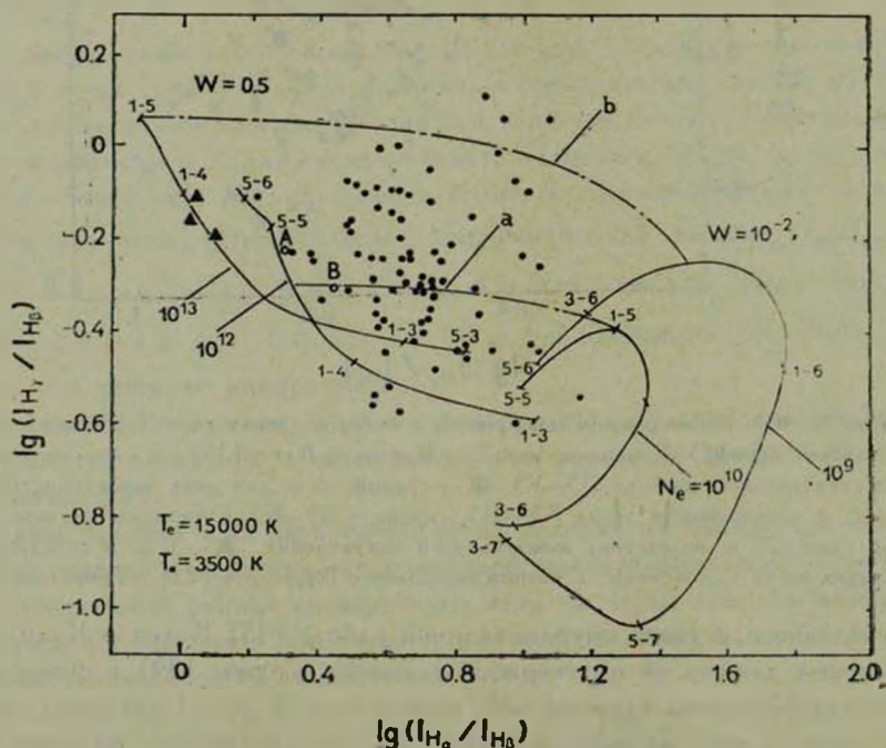
Рис. 2. ● — б. д. совокупности звезд спектральных классов K5—M5 по данным [15], ○ — б. д. в случае А и В планетарной туманности. Сплошные линии представляют теоретические б. д. для ряда значений параметров, штрих — пунктирные кривые соответствуют линейной комбинации зон с различной плотностью. ▲ — то же, что и на рис. 1.
