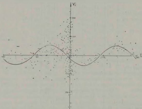
Рис. 2. Распределение пекулярных лучевых скоростей 348 планетарных туманностей V_r , согласно варианту 1 из табл. 1, в зависимости от галактической долготы l'' . Сплошной линией показано теоретическое распределение V_r - l'' , соответствующее этой модели дифференциального галактического вращения с круговыми орбитами для группы объектов, близких к галактической плоскости V_r = A \sin 2(l'' - L) при L'' = 99^\circ , B'' = +20 и V_r = 28.4 км/сек.
