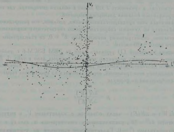
Рис. 1. Распределение наблюдаемых лучевых скоростей 348 планетарных туманностей V_r в зависимости от галактической долготы объекта l'' . Сплошной линией показано теоретическое распределение лучевых скоростей объектов с теми же координатами, точно соответствующее стандартному апексу L'' = 57 , B'' = 22 , V_c = 19.7 км/сек.
