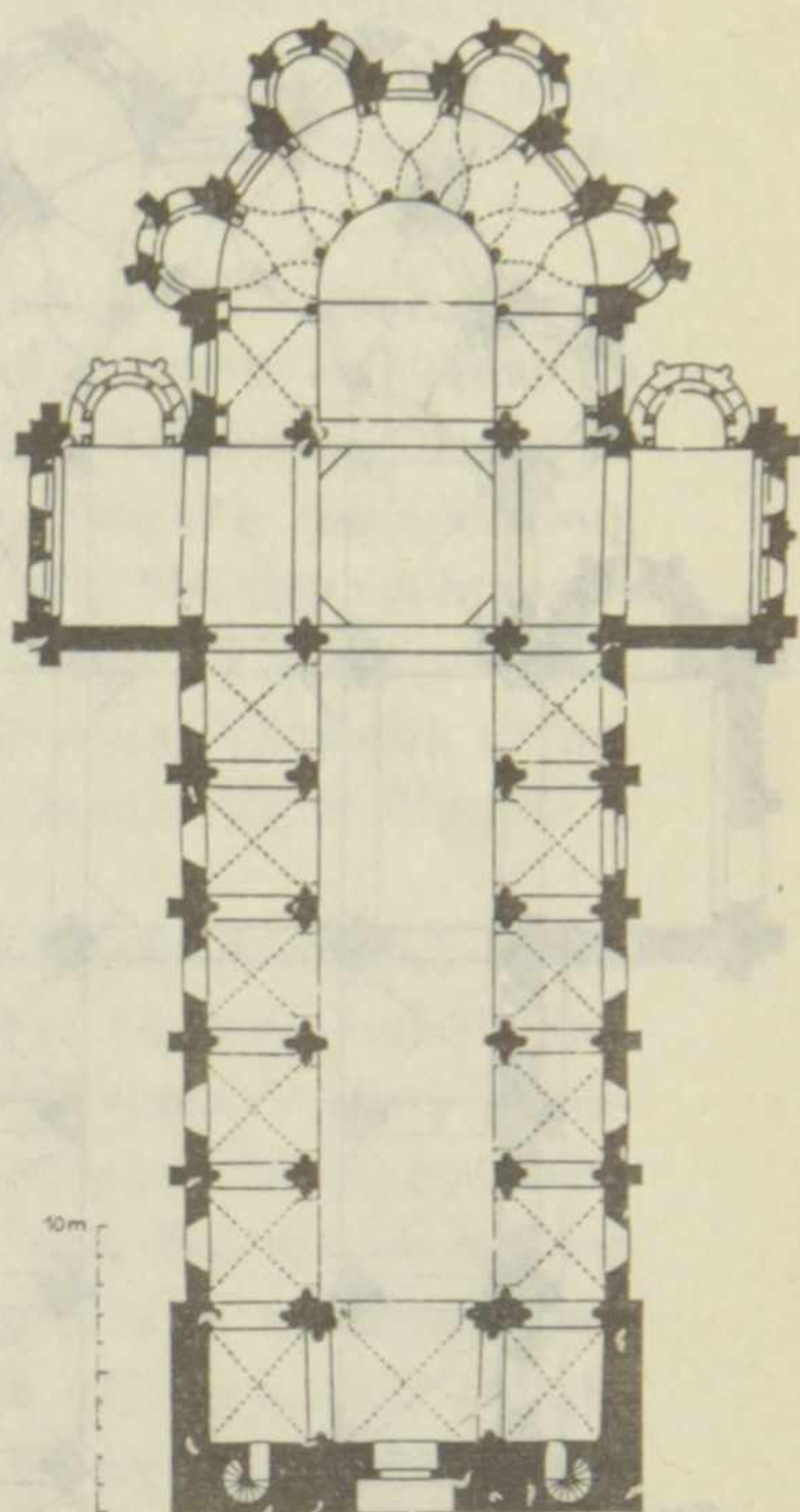
2. ԿԼԵՐՄՈՆ-ՖԵՐԱՆԻ ԱՍՏՎԱԾԱՄՈՐ ԵԿԵՂԵՑՈՒ ՀԱՏԱԿԱԳԻԾԸ
