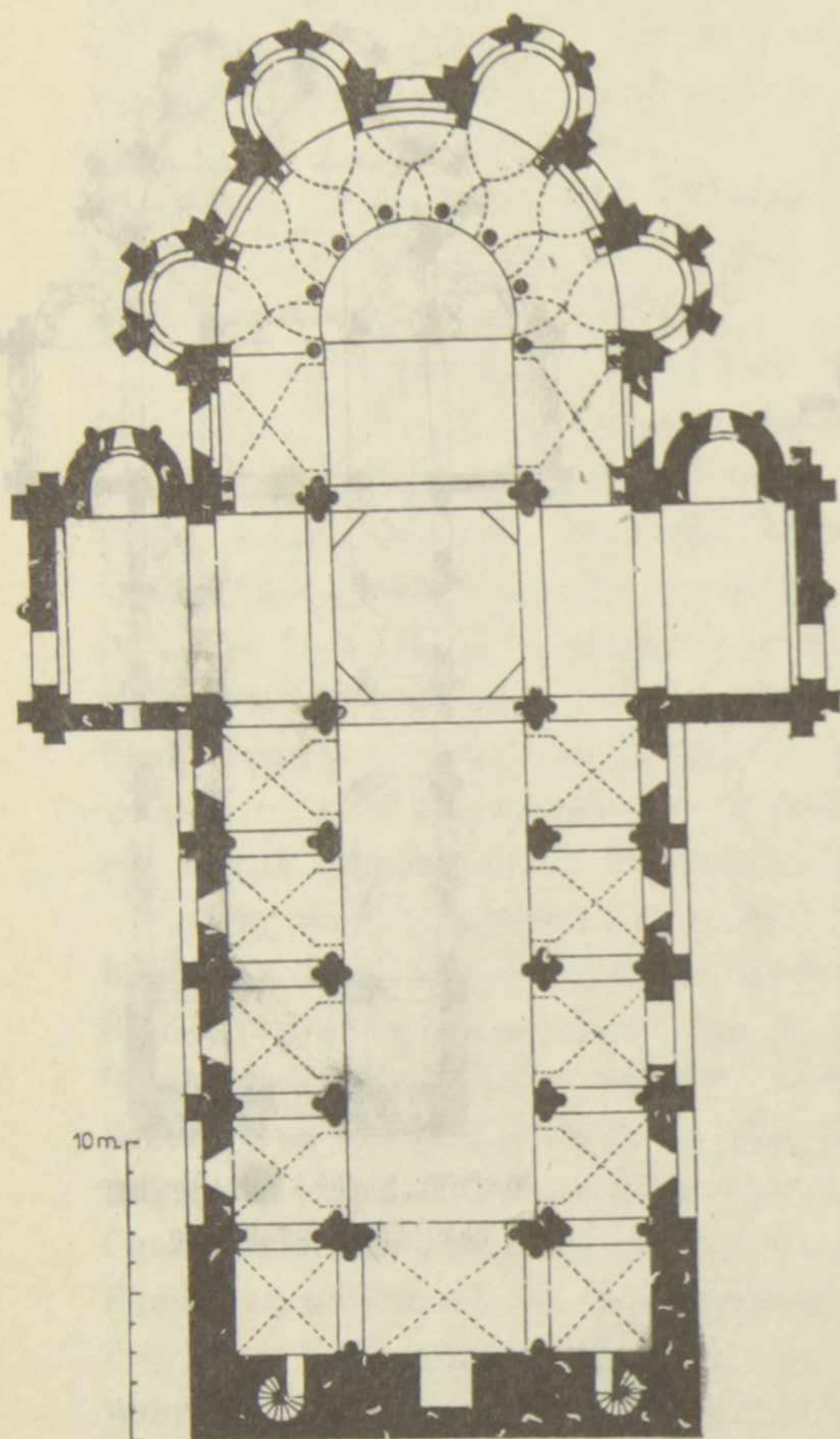
6. ՕՐՍԻՎԱԼԻ ԵԿԵՂԵՑՈՒ ՀԱՏԱԿԱԳԻԾԸ
