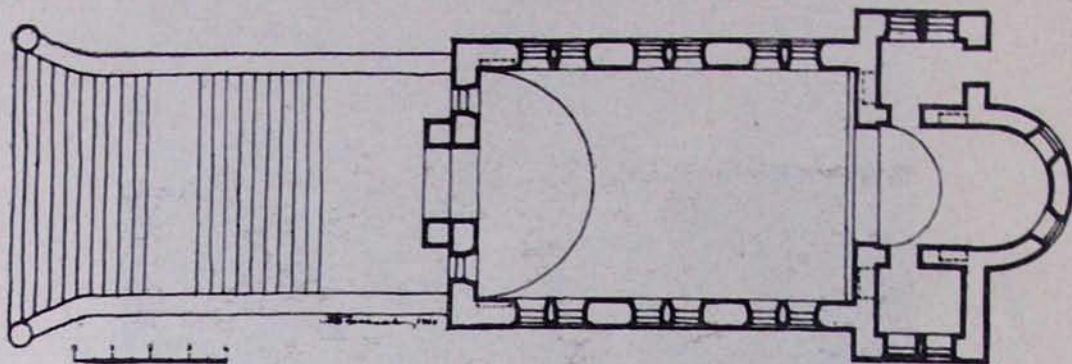
Նկ. 4. Օրինել. հայկական եկեղեցին. հատակագիծ
