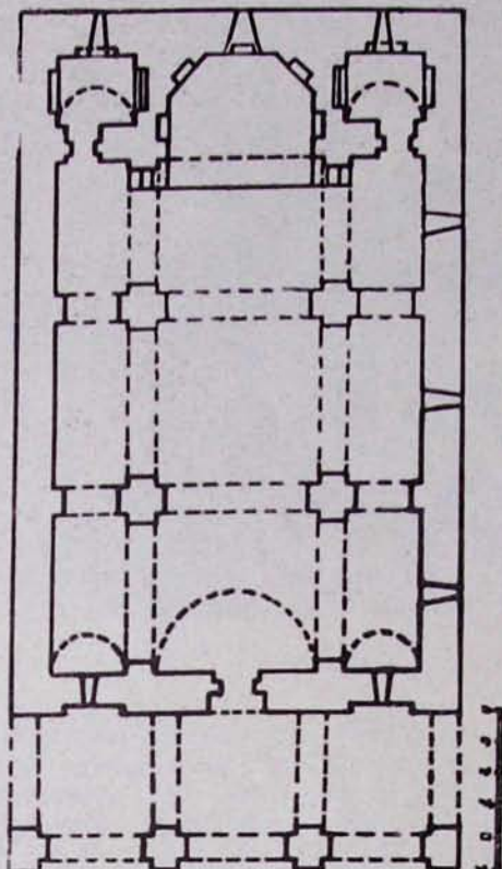
Նկ. 6. Ծրցուի եկեղեցու հատակագիծը
