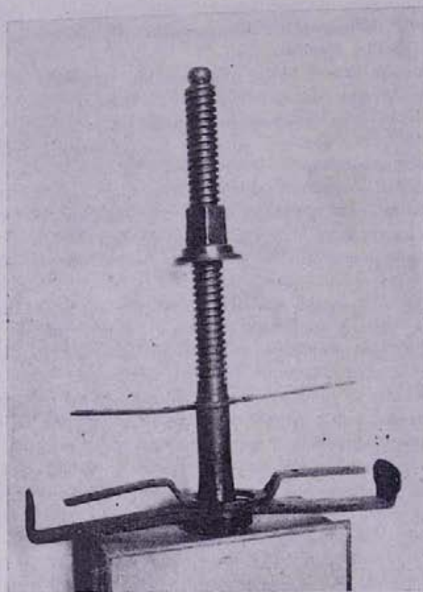
Սիմեոն Երևանցու տպարանում գործածվող փայտայ մամուլի պտտուակը
