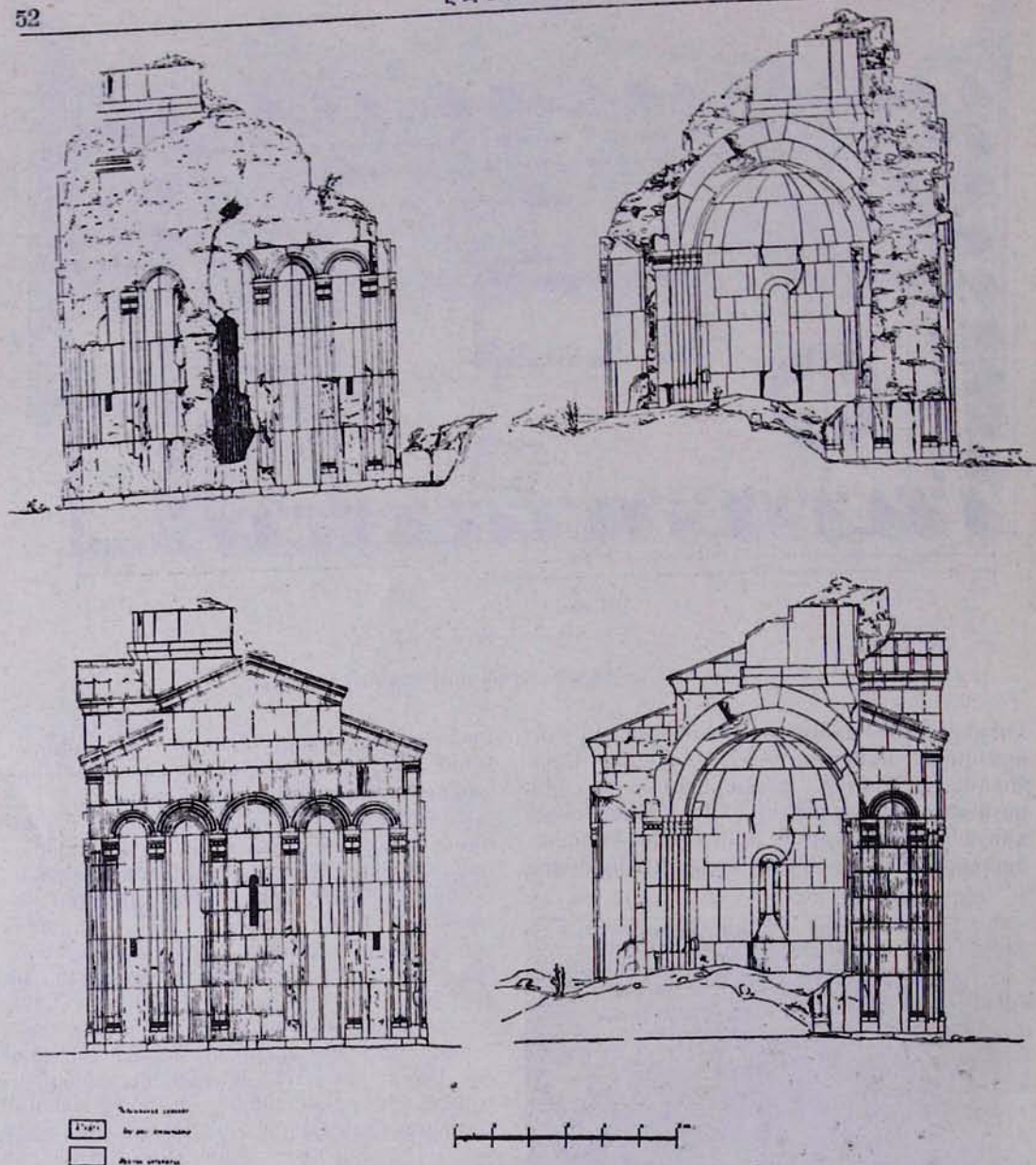
Գծ. № 2. Մարմաշենի երկրորդ եկեղեցու վերանորոգման նախագիծ
