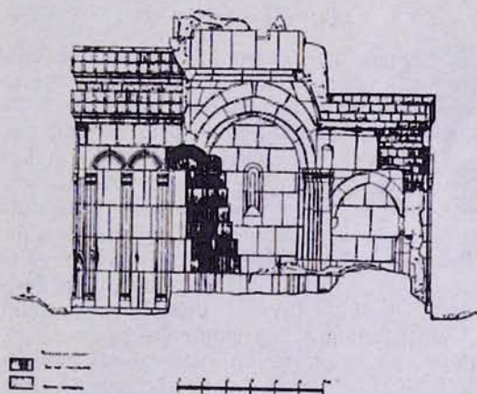
Գծ. № 3. Մարմաշենի երկրորդ եկեղեցու վերանորոգման նախագիծ
