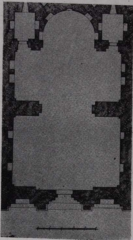
Հավուց թառի վանք.—Նորակառուց անավարտ եկեղեցու հատակագիծը:
