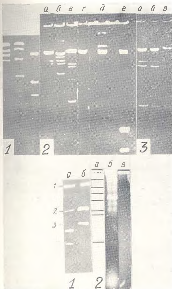
Рис. 1. 1. Электрофоретические профили плазмидных ДНК S. derby K-89 в различных условиях культивирования. 2. Электрофоретические профили плазмидных ДНК S. derby K-89 в составе трансформантов. а), б), в) E. coli J 5-3, трансформированные плазмидными ДНК 1, 2, 3; г) E. coli J 5-3; д) Реп-устойчивый трансформант E. coli J 5-3 (ДНК 3); е) Sm r Str r —устойчивый трансформант E. coli J 5-3 (ДНК 3). 3. Электрофоретические профили плазмидных ДНК экзонуклеотомов S. typhimurium AG-64: а) Реп-устойчивый экзонуклеотант, б) Sm r —устойчивый экзонуклеотант, в) Sm r —устойчивый экзонуклеотант.
