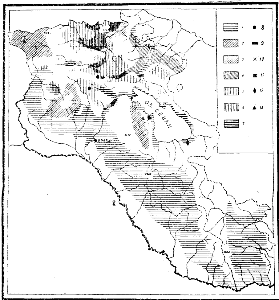
Карта. 1—7—ареалы распространения подвидов скальных ящериц. 1. Lacerta saxicola defilippii (обоюполая форма). 2. Lacerta saxicola valentini . 3. Lacerta saxicola portchinskii . 4. Lacerta saxicola rostombekovi . 5. Lacerta saxicola armeniaca . 6. Lacerta saxicola dahlii . 7. Lacerta saxicola defilippii (партеногенетическая форма). 8—12 — новые находки. 8. L. s. valentini . 9. L. s. portchinskii . 10. L. s. dahlii . 11. L. s. defilippii (партеногенетическая форма). 12. L. s. rostombekovi . 13. L. s. armeniaca .
