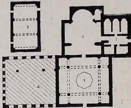
Թեղեկյաց վանքի համալիրը. 1. Կաթողիկե եկեղեցի: 2. Գրատուն-դպրատուն: 3. Առաջին գավիթ (1207): 4. Երկրորդ գավիթ (XIII դ. սկիզբ): 5. Սեղանատուն (XIII դ. սկիզբ): Չափազրությունը՝ Վ. Պետրոսյանցի
