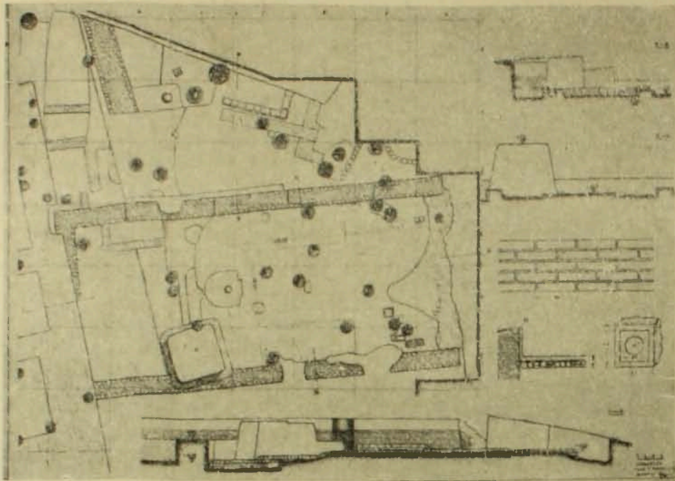
Նկ. 2. Գաշասրահի ընդհանուր հատակագծեր
