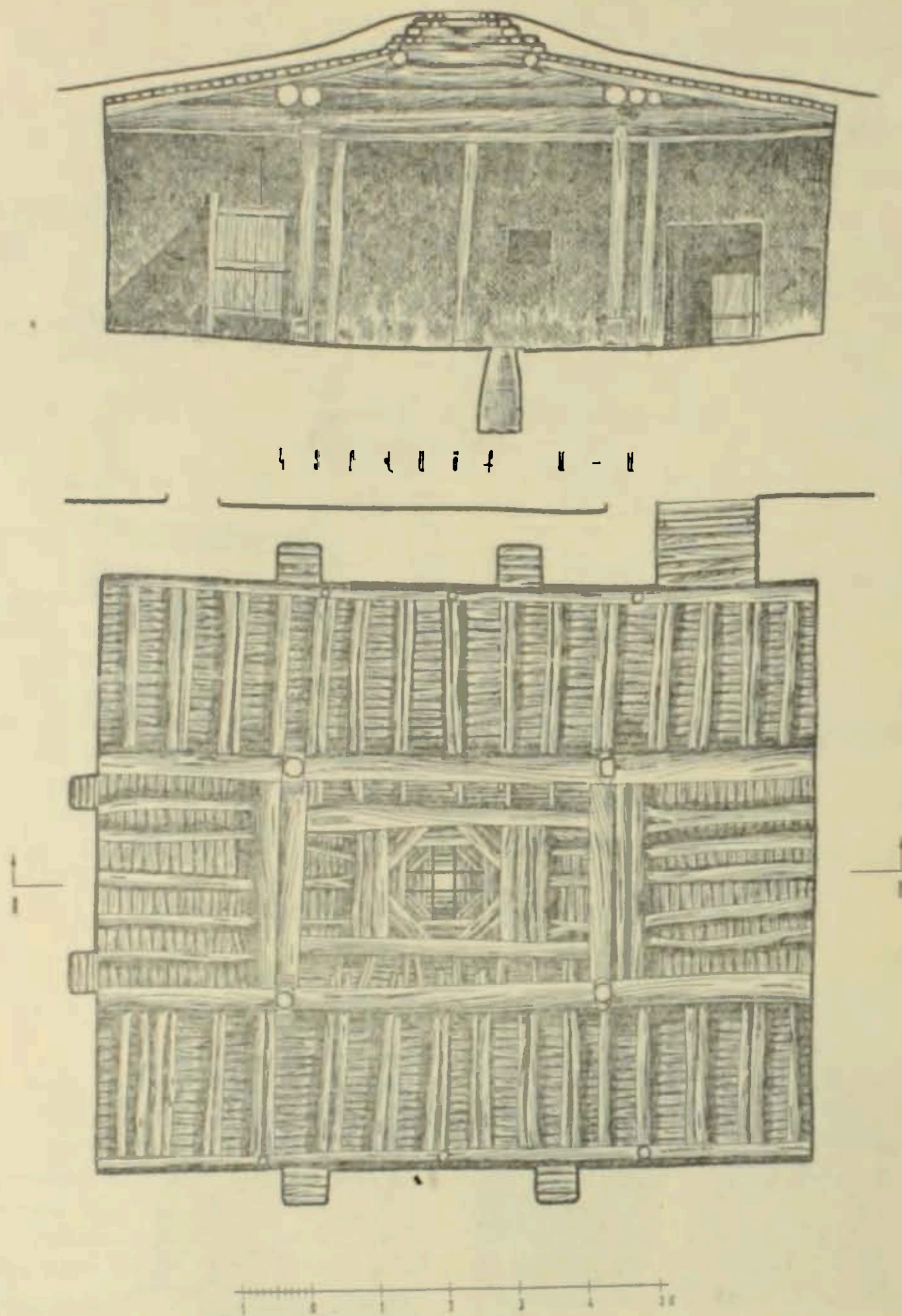
Նկ. 3. Մելիք-Ջաքարյանների տան առաստաղն ու կտրվածքը
