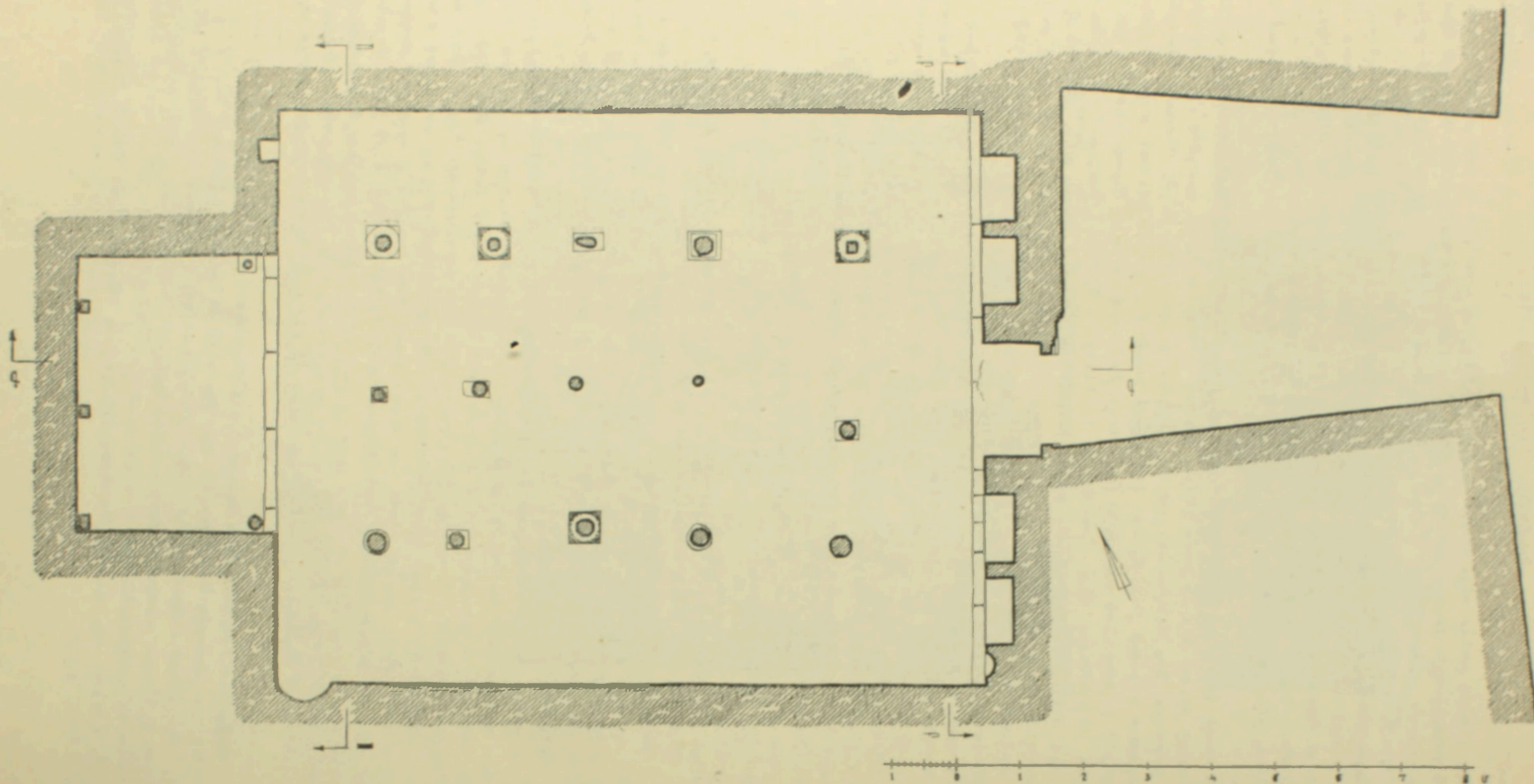
Նկ. 4. Հորս գյուղի «Մեհրախան» տան հատակագիծը
