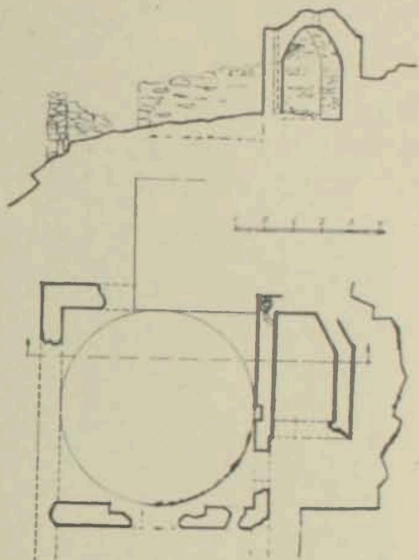
Նկ. 10. Փոքր բաղնիք. հատակագիծ և կտրվածք
