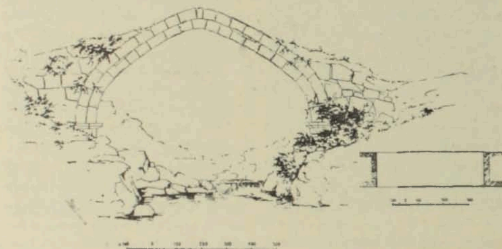
Նկ. 5. Կամուրջ Միսիսանա գետի վրա
