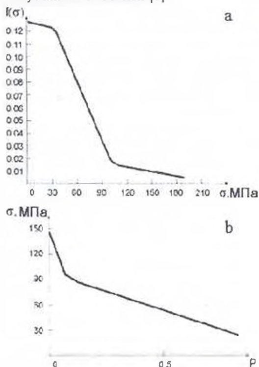
Фиг. 2 Функция плотности (а) и функция нормального распределения (б), построенные при \sqrt{(\sigma^2)} = 60 \text{ МПа} .
