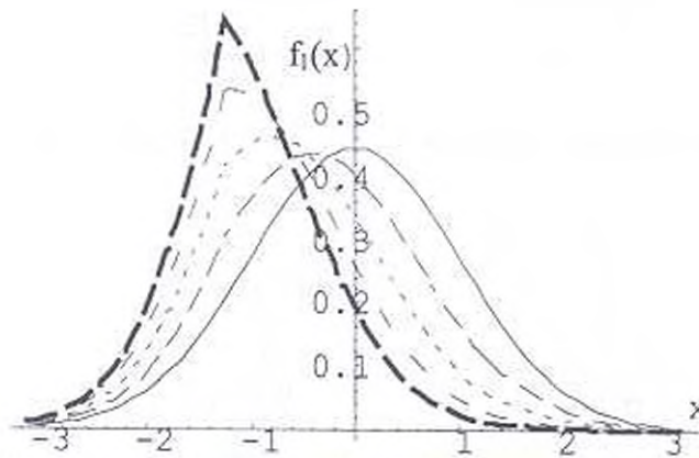
Фиг. 3. Функция плотности распределения при различных значениях n .
