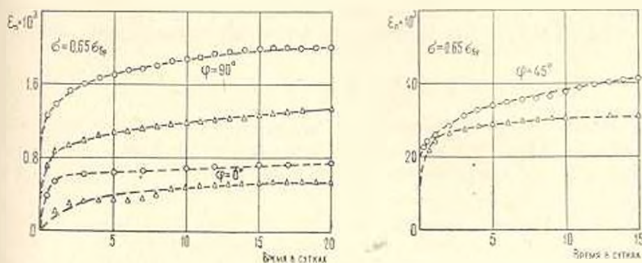
Фиг. 4. Кривые ползучести стеклотекстолита под \sigma = 0.65 \sigma_b : а) при \varphi = 0 и 90^\circ ; б) при \varphi = 45^\circ . \circ — контрольные образцы; \triangle — рабочие образцы.
