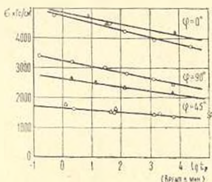
Фиг. 2. Кривые длительной прочности. \circ — контрольные образцы, \triangle — рабочие образцы.
