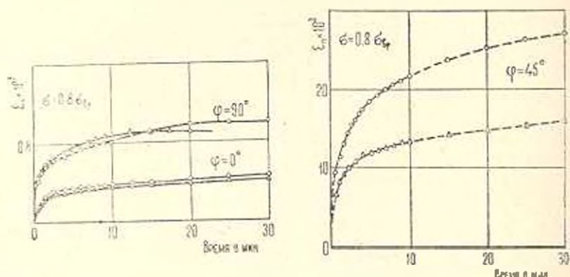
Фиг. 3. Кривые ползучести стеклотекстолита под \sigma = 0.8 \sigma_B : а) при \varphi = 0^\circ и 90^\circ ; б) при \varphi = 45^\circ . \circ — контрольные образцы; \Delta — рабочие образцы.
