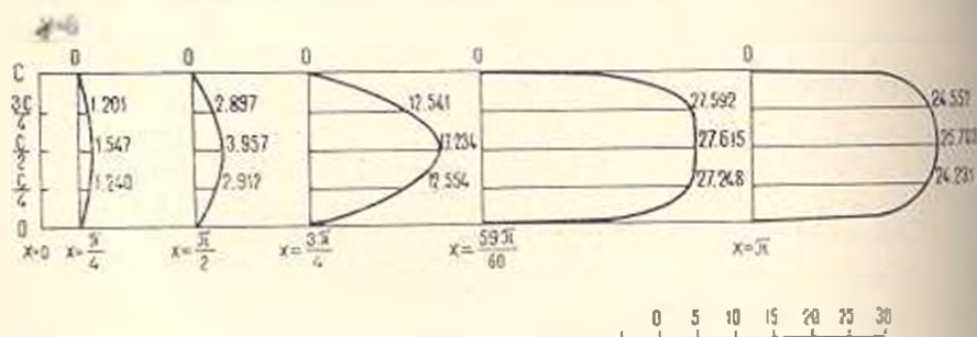
Фиг. 2 Эпюры касательных напряжений \tau_{xz} a = b = 3c = \pi
