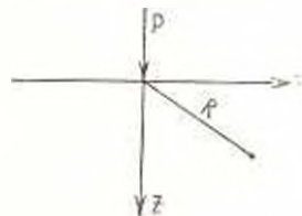
Фиг. 1. Схема к расчету напряженного состояния полупространства при действии на его границе сосредоточенной вертикальной силы P .
