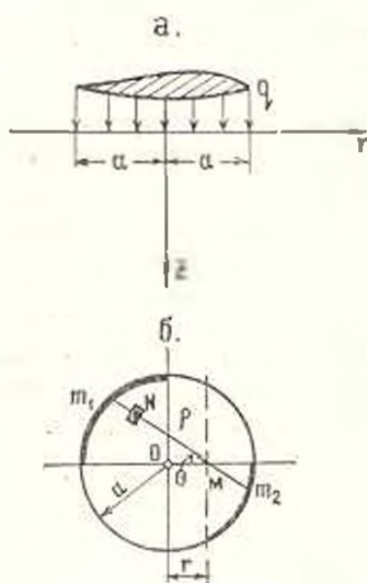
Фиг. 3. Схема к расчету осадки фундаментов при действии равномерно-распределенной нагрузки по площади круга.
