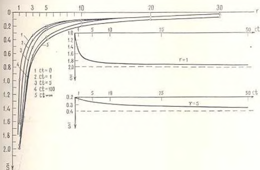
Фиг. 2. Графики приведенных смещений границы полупространства \bar{S}(t) = \frac{S(t)}{P} при действии сосредоточенной силы P при Q(t)=0 и \gamma=0 .
