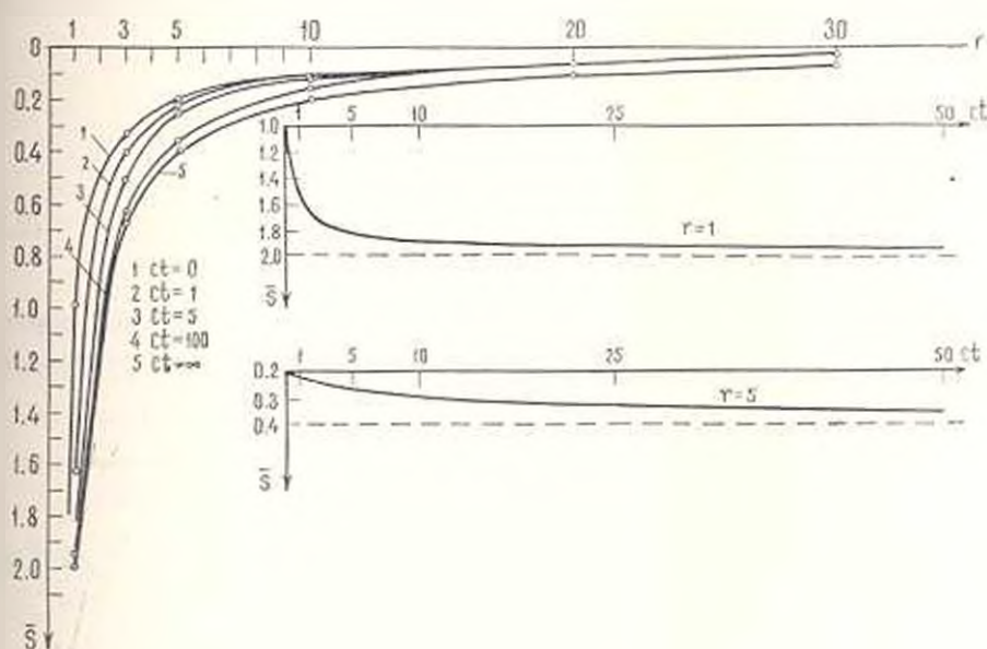
Фиг. 2. Графики приведенных смещений границы полупространства S(t) и S(t)/P при действии сосредоточенной силы P при Q(t)=0 и \gamma_{сх}=0 .
