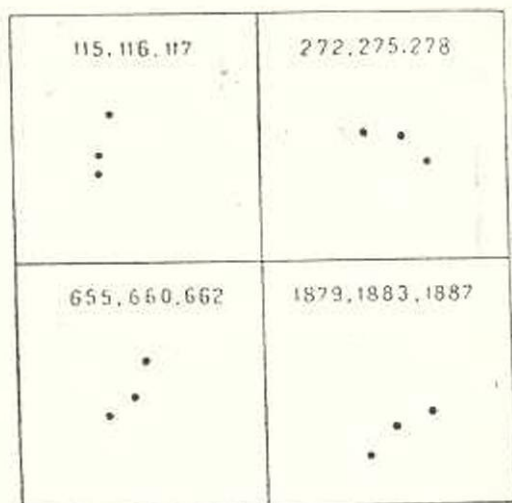
Рис. 3. Четыре наиболее тесные системы из каталога Эймса. Расстояние между компонентами не превосходит 0',8 . Цифры означают номера составляющих галактик по каталогу Эймса.
