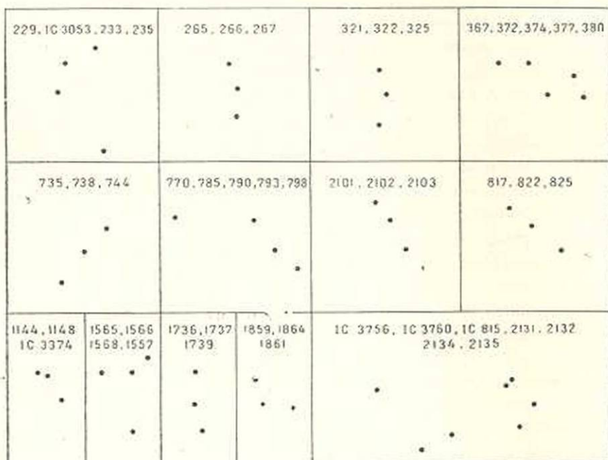
Рис. 4. 13 систем из каталога Эймс, для которых расстояния между компонентами находятся в пределах 0',9-1',3 . Цифры означают номера составляющих галактик по каталогу Эймс.
