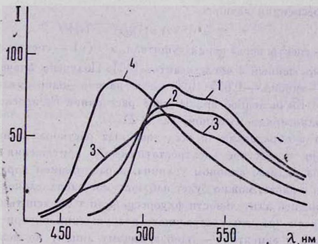
Рис. 2. Спектры флуоресценции: концентрация C = 2,55 \cdot 10^{-5} моль л ^{-1} ; 1 — pH = 4,0 ; 2 — pH = 3,2 ; 3 — 2 N H_2SO_4 ( 0,2 < pH < 1 ); 4 — 5 N H_2SO_4 .
