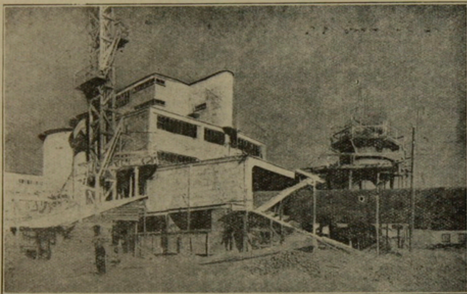
Կառուցուելու վրայ եղող «Ցիմենտի» գործարան, Դավալուի մէջ
