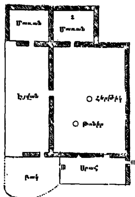
Ձև 28. Մեղրի գիւղէն տան մը յատակագիծը:
