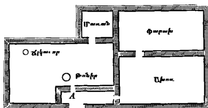
Ձև 30. Ալաշկերտի գաւառէն տան մը յատակագիծը:
